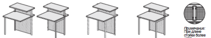
Стойка банковская P/СБ-80МК-120МК левая (правая) Размер: 800/1000/1200x750x1165
