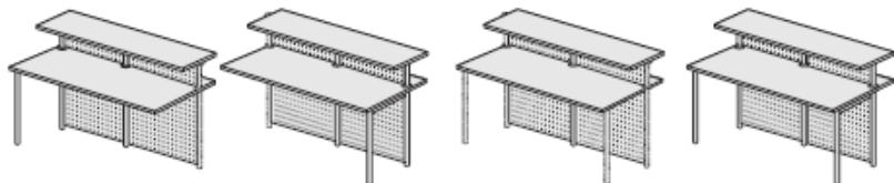
Стойка банковская P/СБ-140МК левая (правая) Размер: 1400x750x1165
